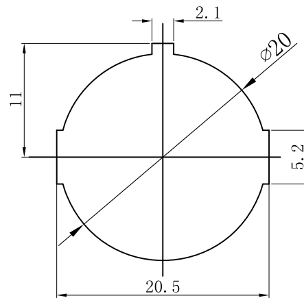
安装面板尺寸 PANEL CUT-OUT
