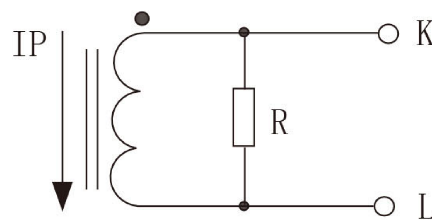
内置取样电阻 电压输出型
