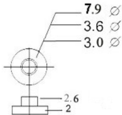
TO-3
